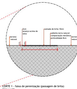
CORTE 1 - faixa de perenização (passagem de brita) ESCALA 1:100
